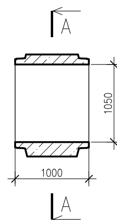
PRZEKRÓJ PODŁUŻNY RURA BOSY-BOSY
