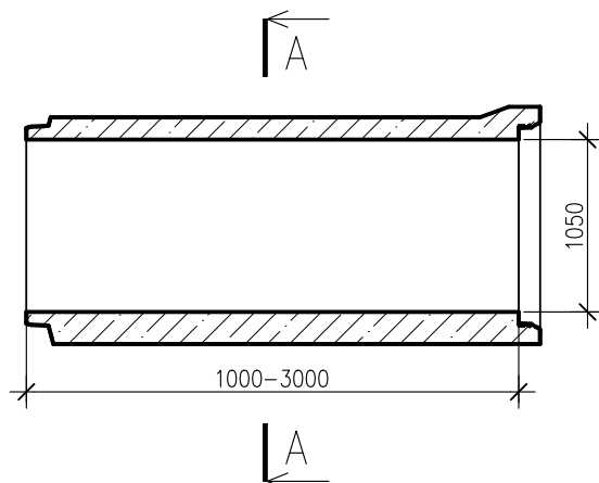
PRZEKRÓJ PODŁUŻNY RURA BOSY-KIELICH
